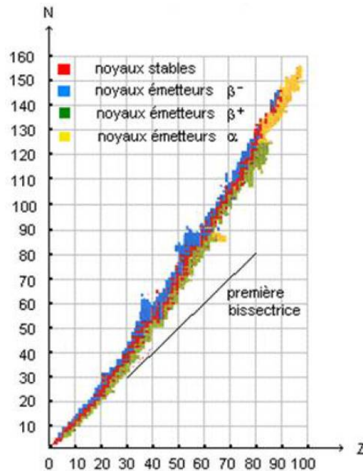
Diagramme de Segré montrant les noyaux stables et les différents types de radioactivités.
