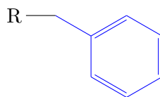
(b) Le groupe benzyle -Bn
