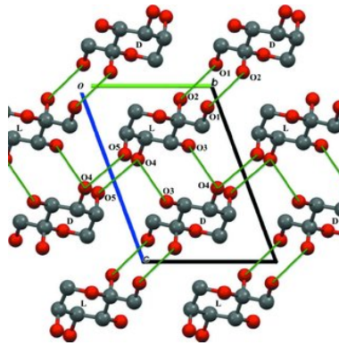
(b) Le fructose
