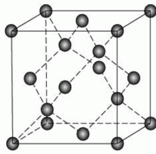
(a) Le diamant
