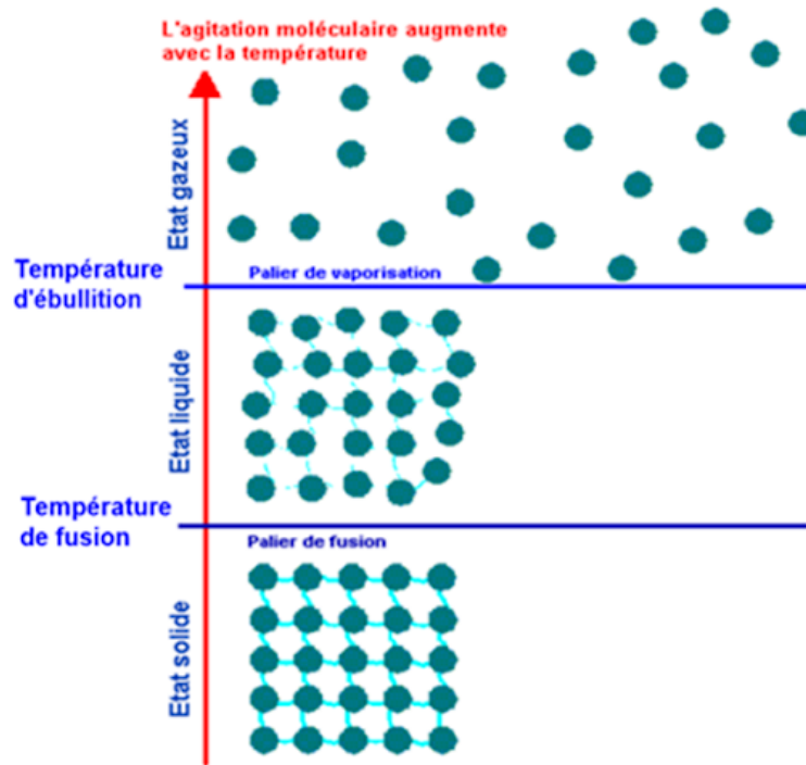
Les différentes représentations des états de la matière à l'échelle microscopique.
