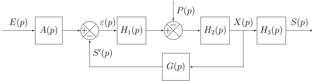
FIGURE 26 – Schéma-blocs minimal d'un système asservi.
