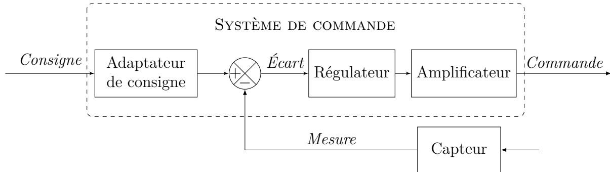
FIGURE 5 – Structure générique d'un système de commande.
