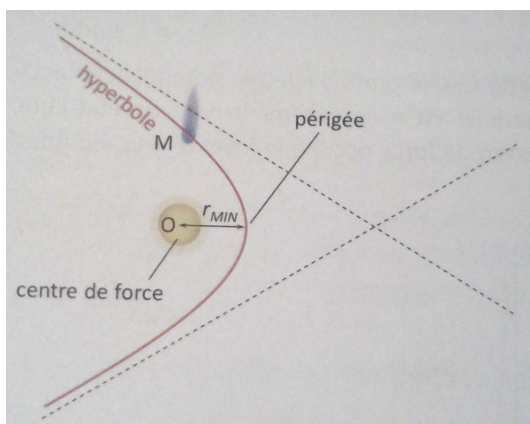
FIGURE 4 – Si son énergie mécanique est positive, le système soumis à une force newtonienne attractive décrit une branche d'hyperbole dont le centre de force occupe le foyer le plus proche.
