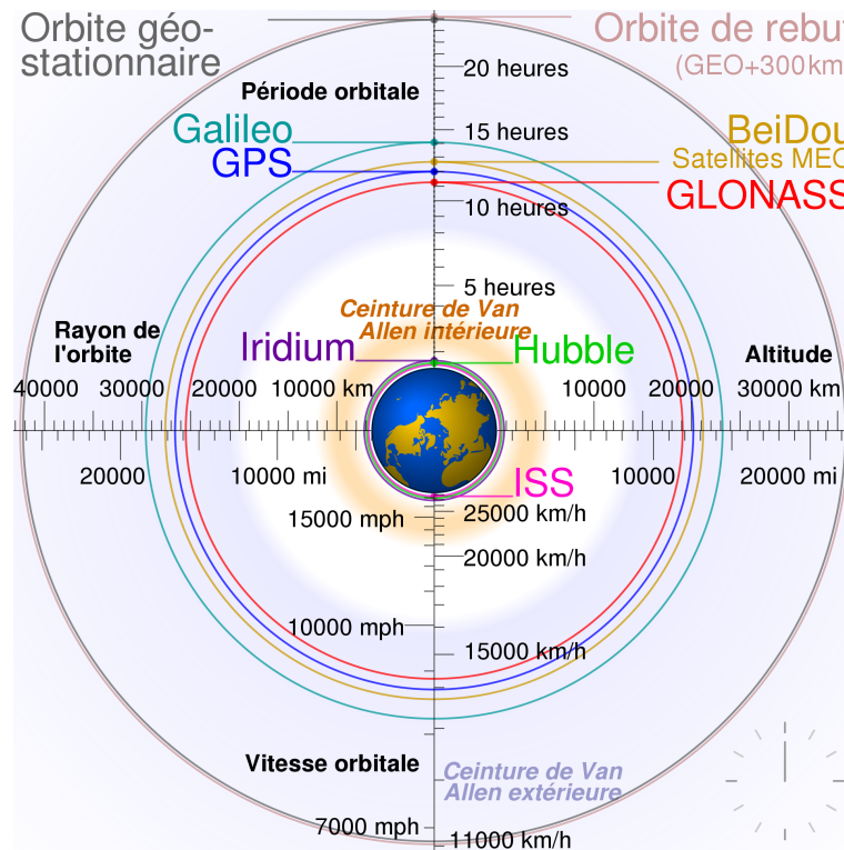
FIGURE 7 – Schéma à l'échelle montrant la Terre, les principales orbites (orbites basse, moyenne et géostationnaire) utilisées par les satellites, les vitesses et les périodes orbitales à différentes altitudes ainsi que la position de quelques satellites ou constellations de satellites remarquables : GPS, GLONASS, Galileo and Compass, Station spatiale internationale, télescope Hubble et la constellation Iridium (Par cmglee - Travail personnel, CC BY-SA 3.0, https://commons.wikimedia.org/w/index.php?curid=16891766 )
