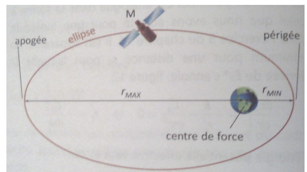
FIGURE 5 – Si son énergie mécanique est négative, le système soumis à une force newtonienne attractive décrit une ellipse dont le centre de force occupe l'un des foyers.
