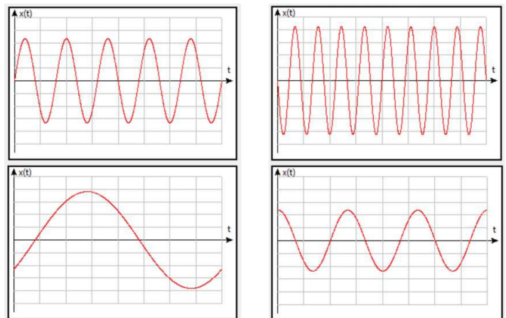
Fig. 1 Quatre acquisitions de la position x(t) d'un oscillateur harmonique en fonction du temps.
