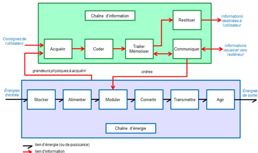
FIGURE 3 – Chaîne d'information et de puissance à compléter
