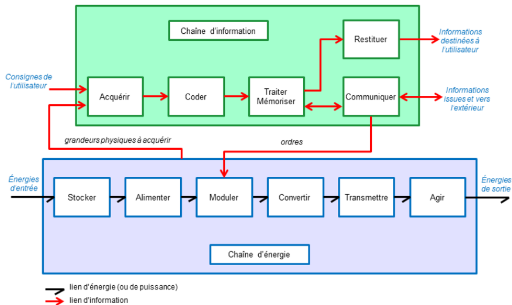
FIGURE 4 – Chaîne d'information et de puissance à compléter
