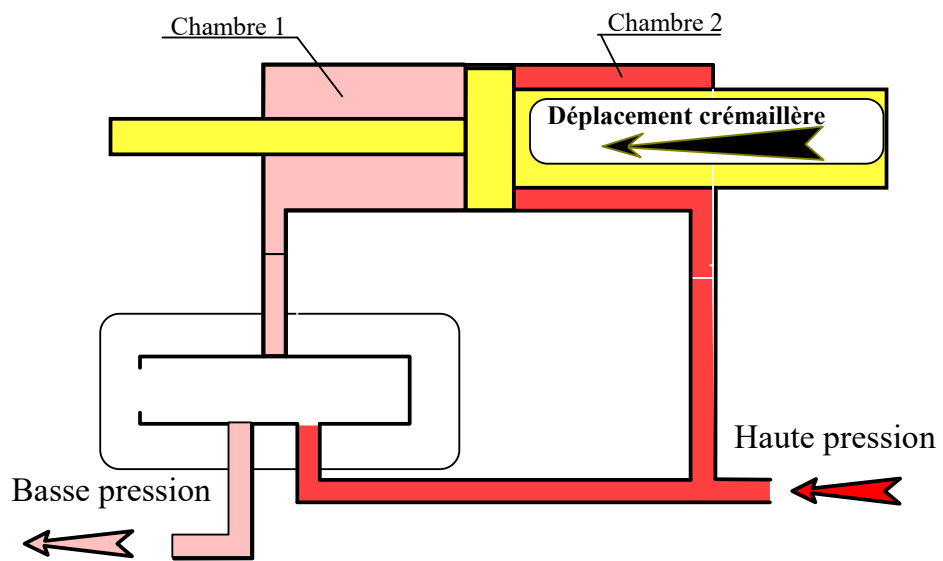
Figure c : Phase de braquage dans l'autre sens
