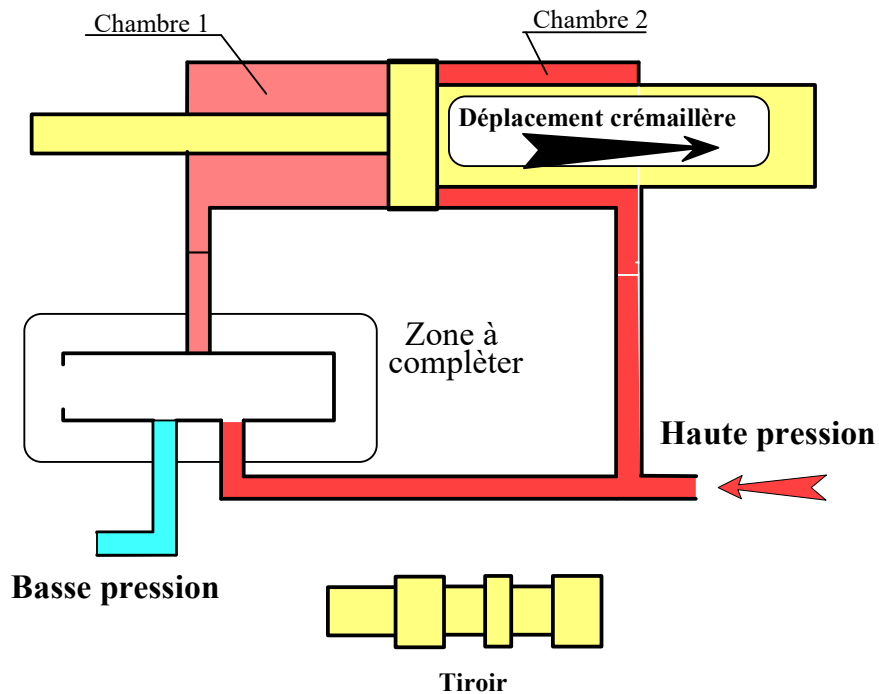
Figure b : Phase de braquage
