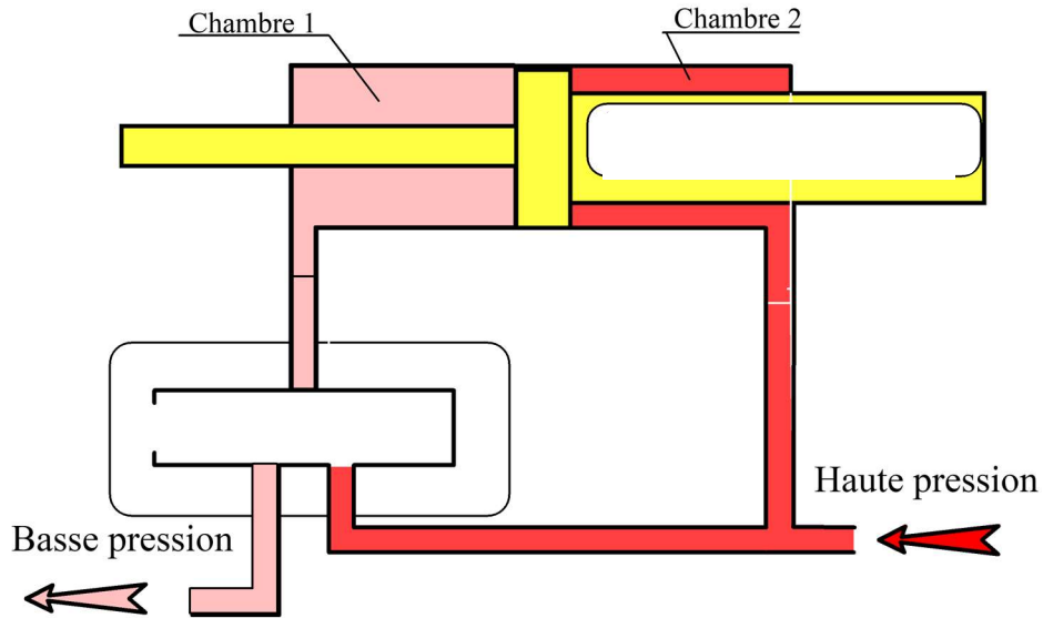
Figure b : Phase de braquage
