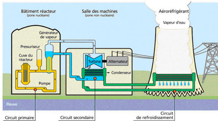
FIGURE 1 : Architecture du circuit de production d'énergie électrique dans une centrale nucléaire
