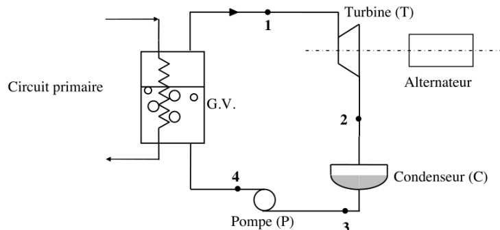
Figure 1 : circuit secondaire simplifié
