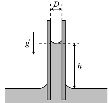
Figure 1 : Le fluide monte dans un tube de section D et sa surface libre forme un ménisque incurvé vers le bas
