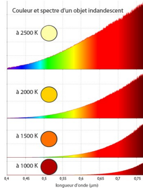
Spectres de sources incandescentes en fonction de leur température.
