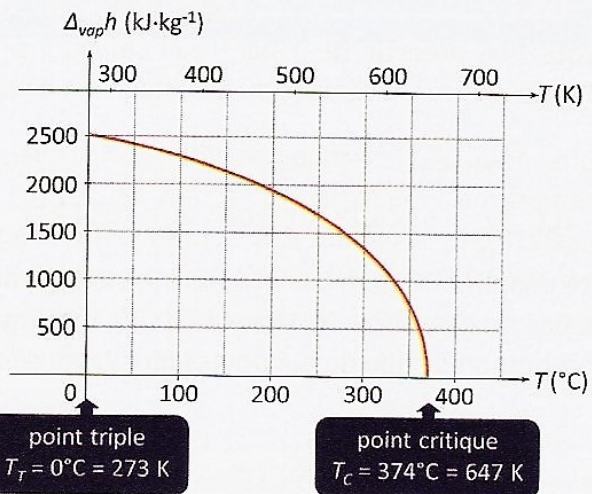
Fig 36. Évolution de l'enthalpie de vaporisation de l'eau avec la température (chaleur latente). Elle est définie entre le point triple et le point critique, pour lequel elle s'annule.
