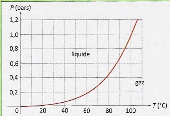
Fig 37. Courbe de saturation de l'eau entre 0°C et 100°C.
