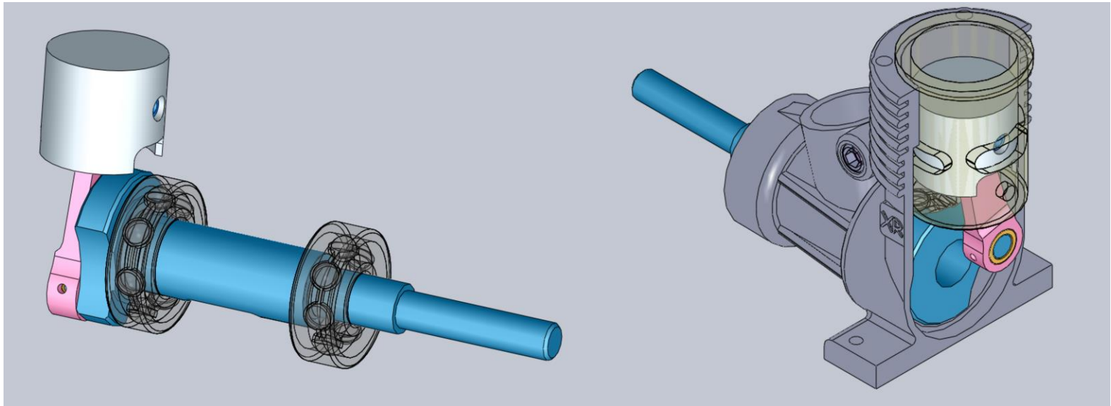
Vue en perspective sans corps du moteur et sans chemise
