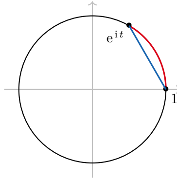
FIGURE 3 – |e^{it} - 1| représente la longueur du segment d'extrémités 1 et e^{it} . Ce segment est en bleu , |t| représente la valeur absolue de l'angle de e^{it} donc la longueur de l'arc, cet arc est en rouge . Comme la ligne droite est le plus court chemin qui relie deux points, |e^{it} - 1| \leq |t|
