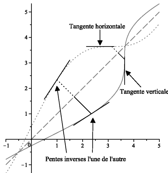
FIGURE 4.3 – Dérivées d’une bijection et de sa réciproque
