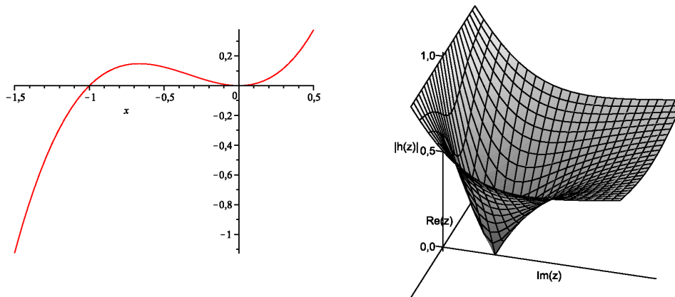
(a) Fonction g de l'exercice 1.23
