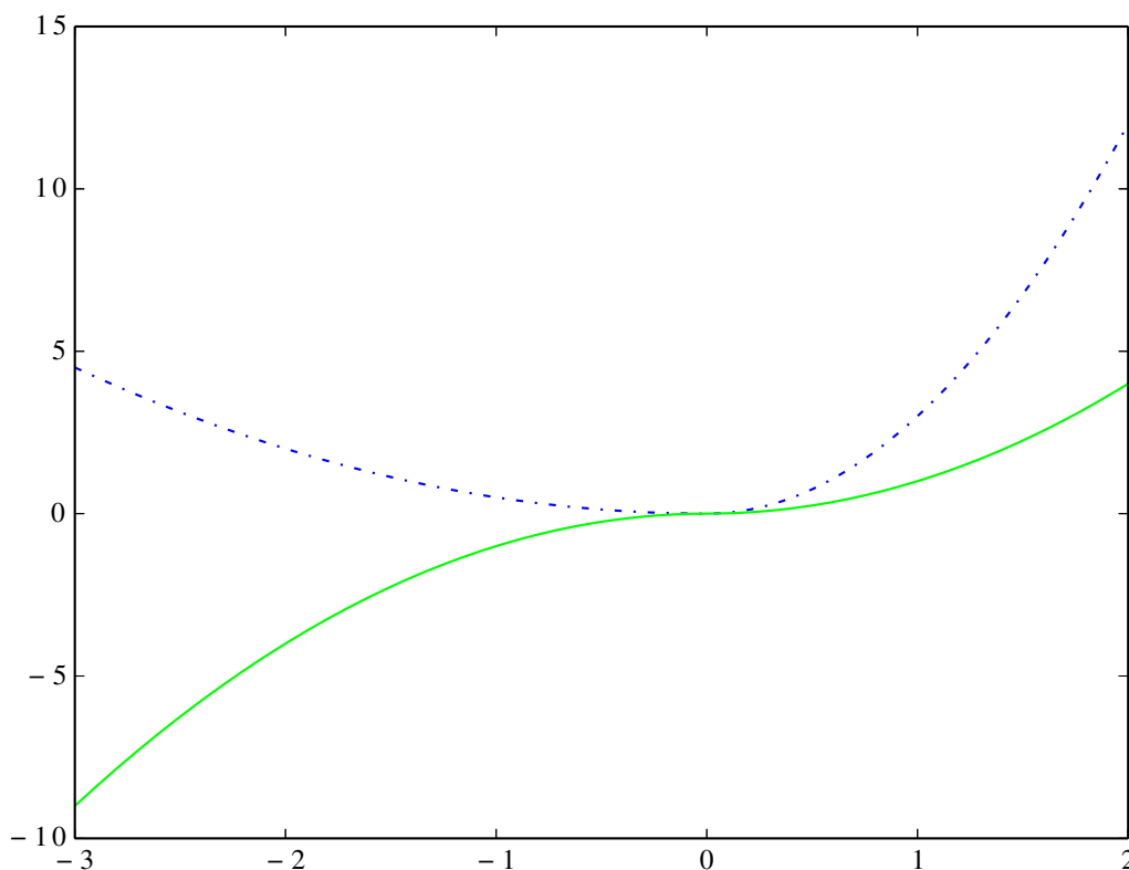
Deux solutions : en pointillés, \lambda_1 = 3, \lambda_2 = \frac{1}{2} , en trait plein, \lambda_1 = 1, \lambda_2 = -1 .
