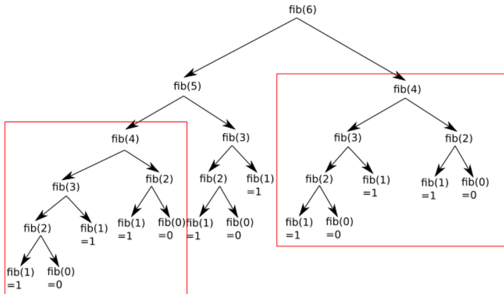
FIGURE 1 – Illustration de l'appel de fib(6)
