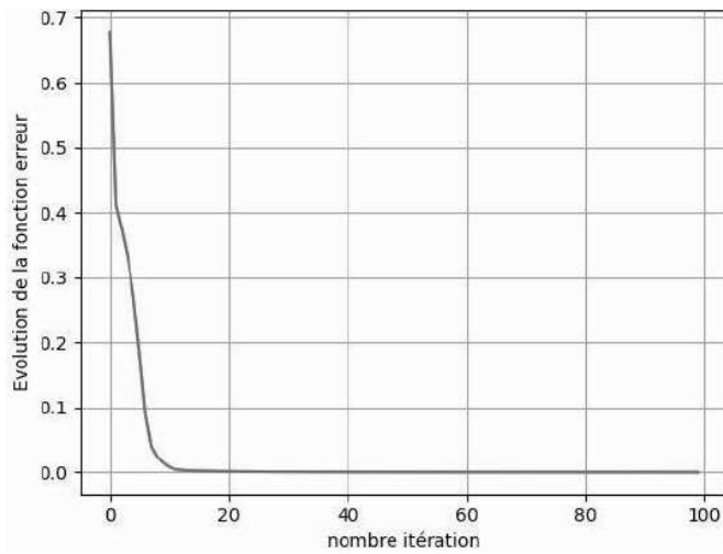
Figure 19 - Entraînement modèle
