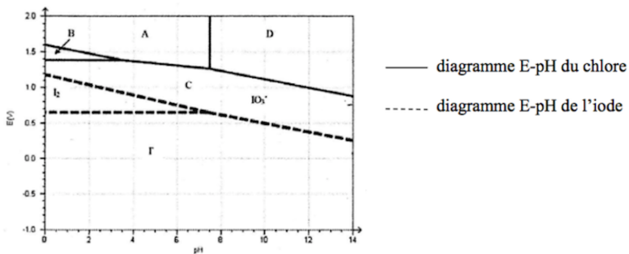
Figure 19 - Diagrammes E-pH du chlore et de l'iode
