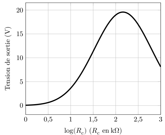
(b) Tension de sortie
