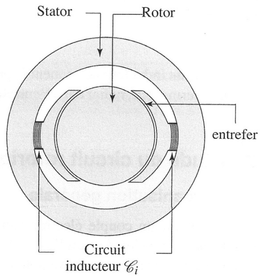
Figure 27.1 – Description de la machine à courant continu.
