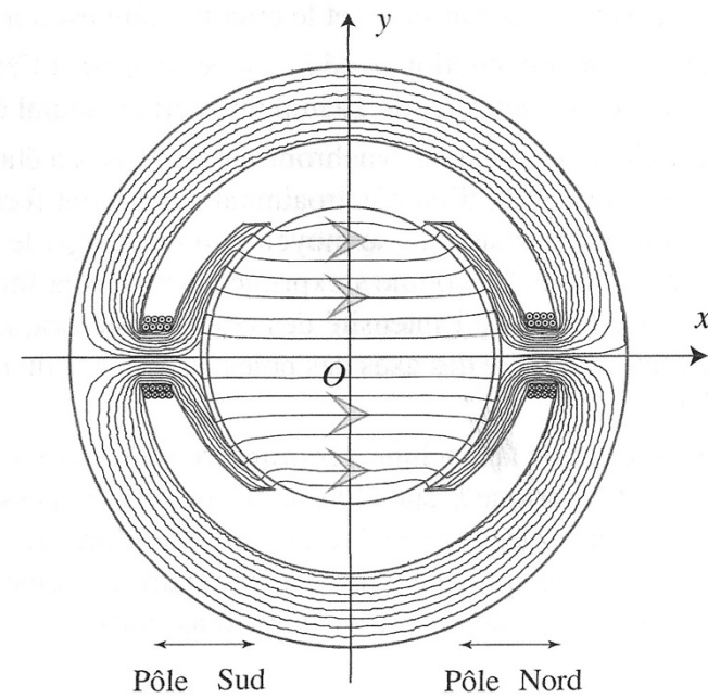
Figure 27.2 – Carte du champ magnétique inducteur.
