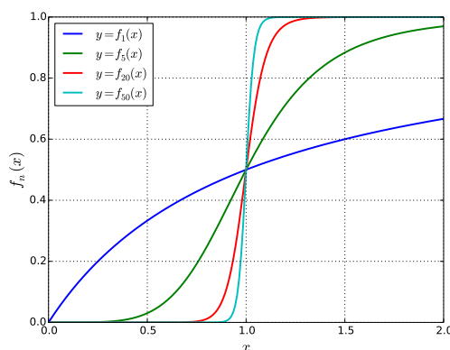
FIGURE 1 — \frac{x^n}{1+x^n} pour n \in \{1, 5, 20, 50\}
