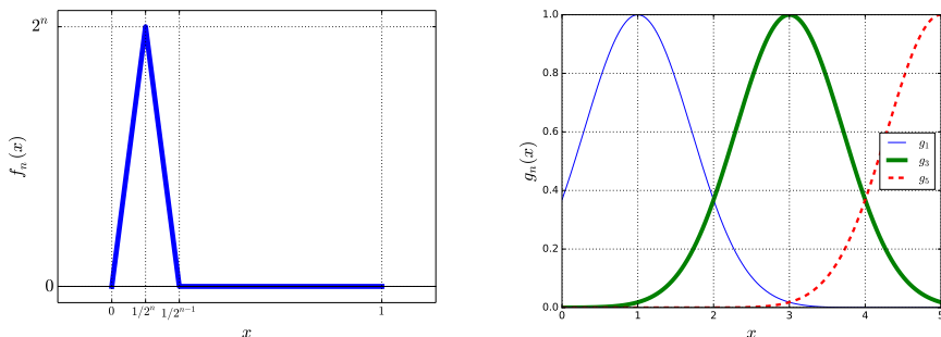
FIGURE 4 – Chapeau pointu et bosse glissante
