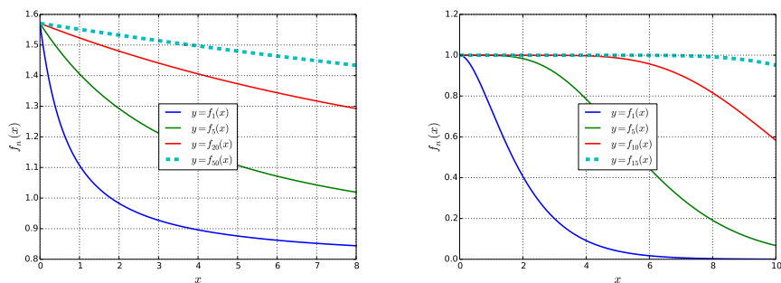
FIGURE 2 – \text{Arctan} \frac{n+x}{x} pour n \in \{1, 5, 20, 50\} et e^{-x} \sum_{k=0}^n \frac{x^k}{k!} pour n \in \{1, 5, 10, 15\}
