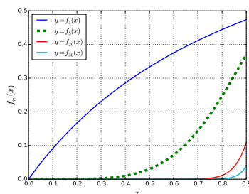
FIGURE 3 – \frac{x^n}{1+x^n} sur [0; 0,9] pour n \in \{1, 5, 20, 30\}
