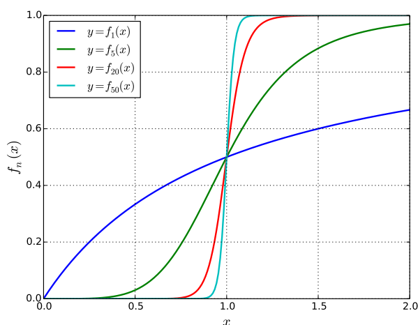
FIGURE 1 — \frac{x^n}{1+x^n} pour n \in \{1, 5, 20, 50\}
