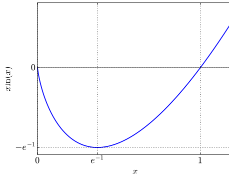
FIGURE 6 – Une fonction usuelle (?)
