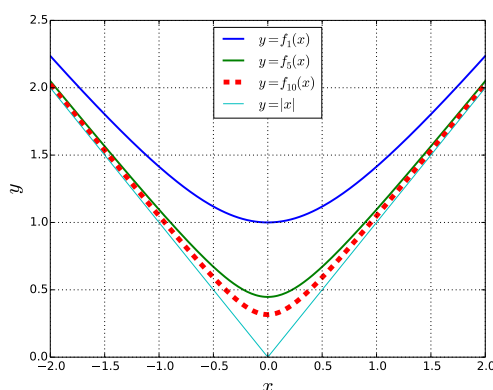
FIGURE 5 – Même avec la convergence uniforme de (f_n)_{n \in \mathbb{N}} , ça ne passe pas
