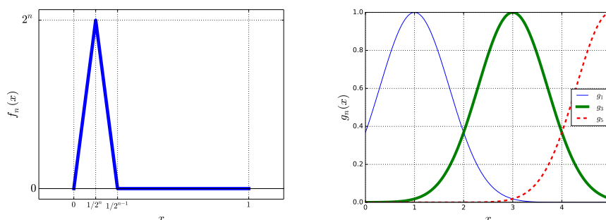
FIGURE 4 – Chapeau pointu et bosse glissante
