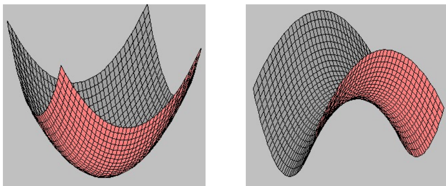
FIGURE 1 – Paraboloïdes elliptique ( z = x^2 + y^2 ) et hyperbolique ( z = x^2 - y^2 )
