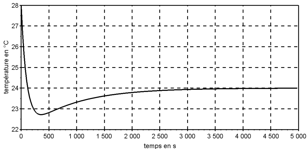
Figure 10 - Résultat simulation finale
