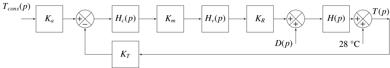
Figure 9 - Schéma-bloc de la commande du système
