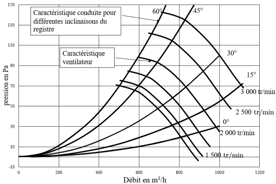
Figure 7 - Caractéristique aérolitique
