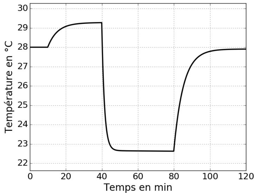
Figure 5 - Simulation de l'évolution temporelle de la température de la pièce
