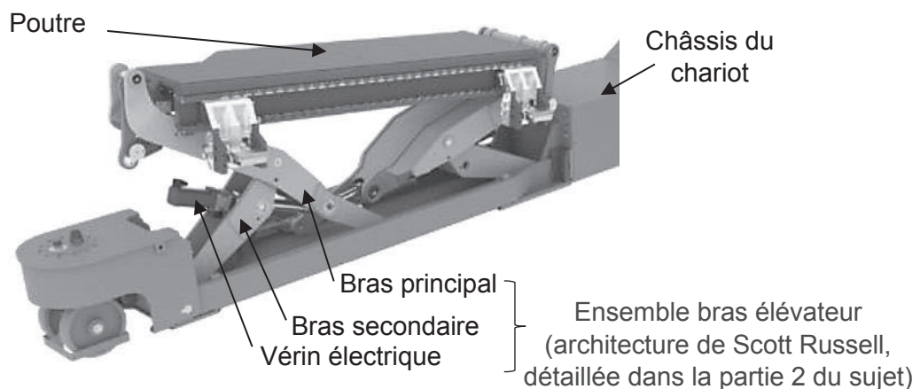
Figure 3 - Ensemble bras élévateur
