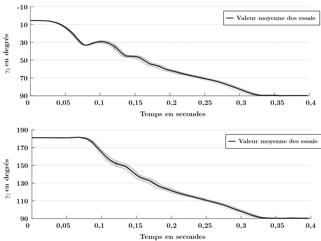
Figure 14 - Relevés des angles \gamma_1 et \gamma_2 pour la phase de dépliement
