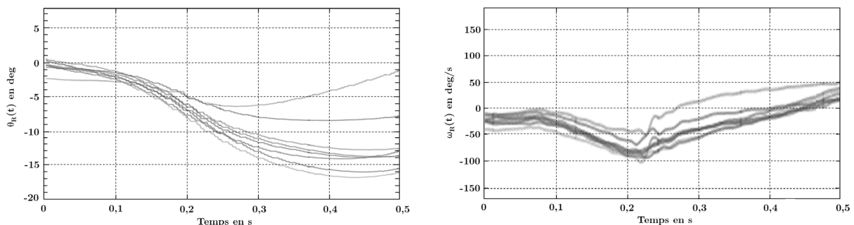
Figure 20 - Évolutions de l'angle de roulis (en degrés) et de la vitesse de rotation en roulis (en deg/s) du drone sont donnée pour 10 essais.
