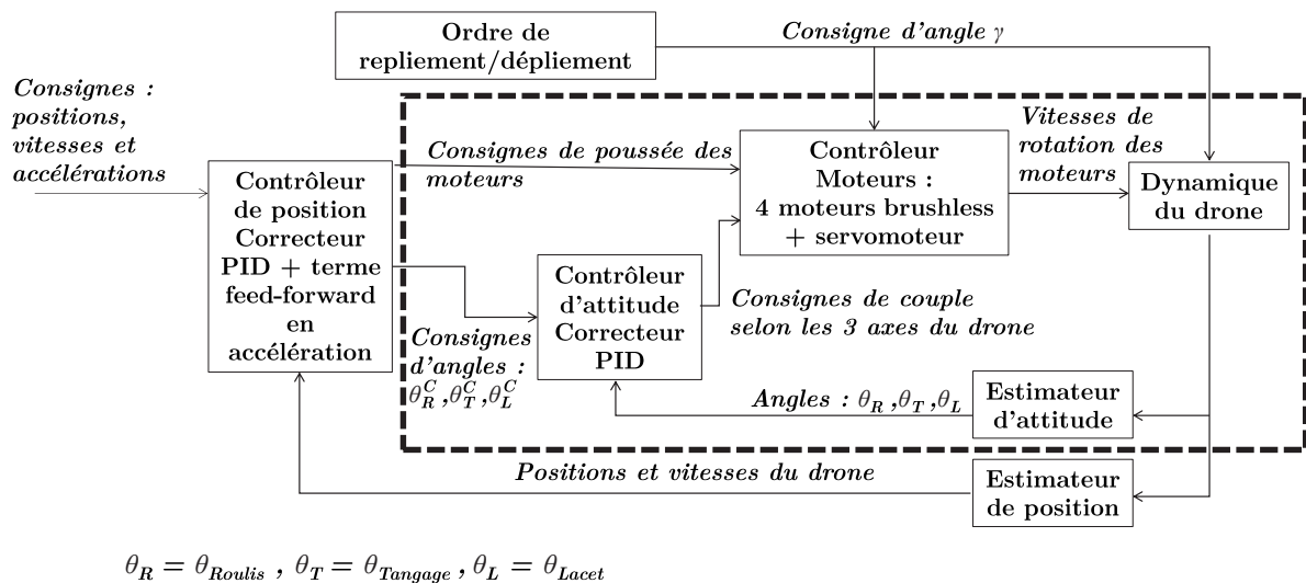
Figure 15 - Structure de commande du drone
