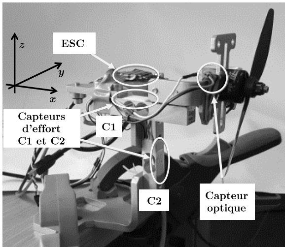
Figure 17 - Vue et schéma du banc d'essai pour déterminer les composantes T et Q de l'action de l'air sur l'hélice en fonction de la vitesse de rotation de l'hélice
