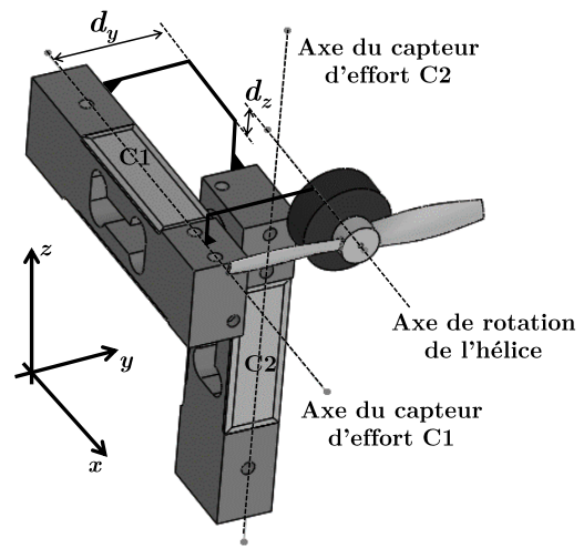
Figure 17 - Vue et schéma du banc d'essai pour déterminer les composantes T et Q de l'action de l'air sur l'hélice en fonction de la vitesse de rotation de l'hélice
