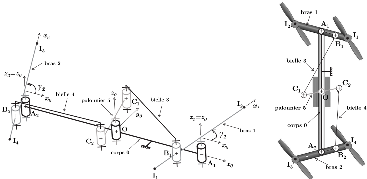
Figure 10 - Modélisation cinématique en perspective et plane en vue de dessus du mécanisme de mise en mouvement des bras du drone basé sur un double système 4 barres
