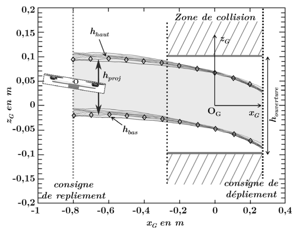
Figure 5 - Vues de dessus et de côté de l'envergure du drone durant huit passages de l'ouverture
