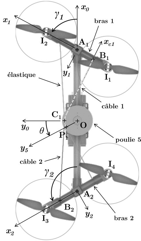
Figure 25 - Mécanisme de mise en mouvement du bras
