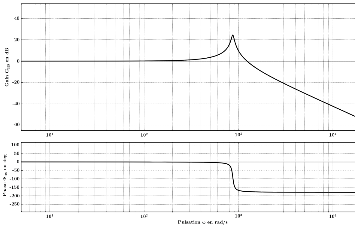
Diagrammes de Bode
