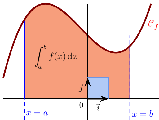
Figure IX.2 – \int_a^b f(x) dx représente l'aire algébrique du domaine orangé en unité d'aire.
