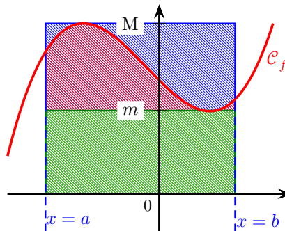
Figure IX.4 – D'un point de vue graphique, l'aire \int_a^b f(x) dx est encadrée par l'aire des deux rectangles inférieur et supérieur. L'intégrale d'une fonction continue sur un intervalle [a; b] ne peut donc faire n'importe quoi comme devenir infinie par exemple. Elle est bornée par le produit des extrema de la fonction par la longueur de l'intervalle.
