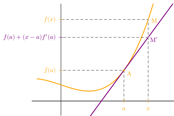
Figure XVI.5 – La tangente est la meilleure approximation affine de f au point a .
