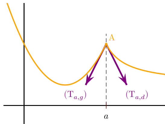
Figure XVI.3 – En un point anguleux, la fonction est continue sans être dérivable.
