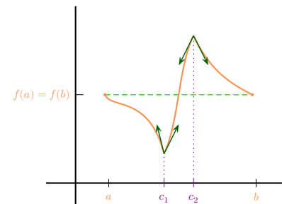
Figure XVI.9 – La dérivabilité est nécessaire.
