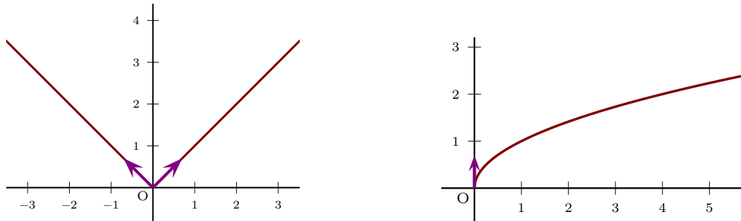
Figure XVI.2 – Les fonctions valeur absolue x \mapsto |x| et racine carrée x \mapsto \sqrt{x} ne sont pas dérivables en 0.
