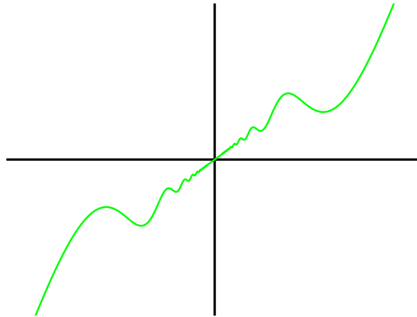
Figure XVI.13 – Une fonction dérivable peut avoir une dérivée strictement positive en un point sans être monotone sur un voisinage de celui-ci.
