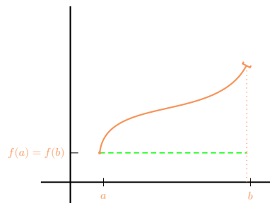
Figure XVI.8 – La continuité est nécessaire.
