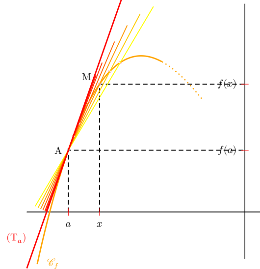
Figure XVI.1 – Tangente à une courbe vue comme limite de ses sécantes.
