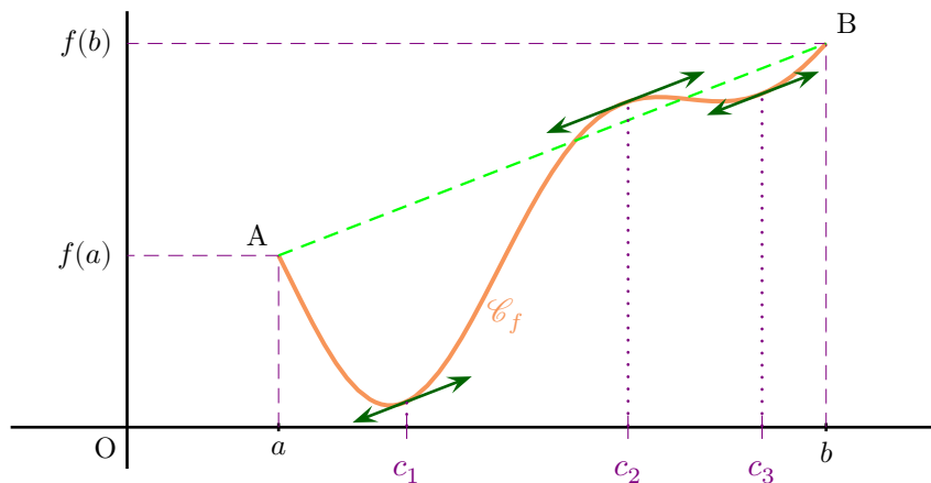
Figure XVI.10 – La courbe d’une fonction dérivable passant par deux points A et B admet une tangente parallèle à la droite (AB) entre ces derniers.
