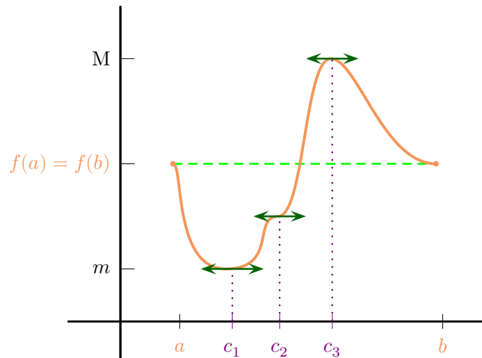
Figure XVI.6 – La courbe d’une fonction dérivable prenant une même valeur en deux points admet une tangente horizontale entre ces derniers.
