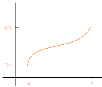
Figure XVI.7 – La condition f(a) = f(b) est nécessaire.
