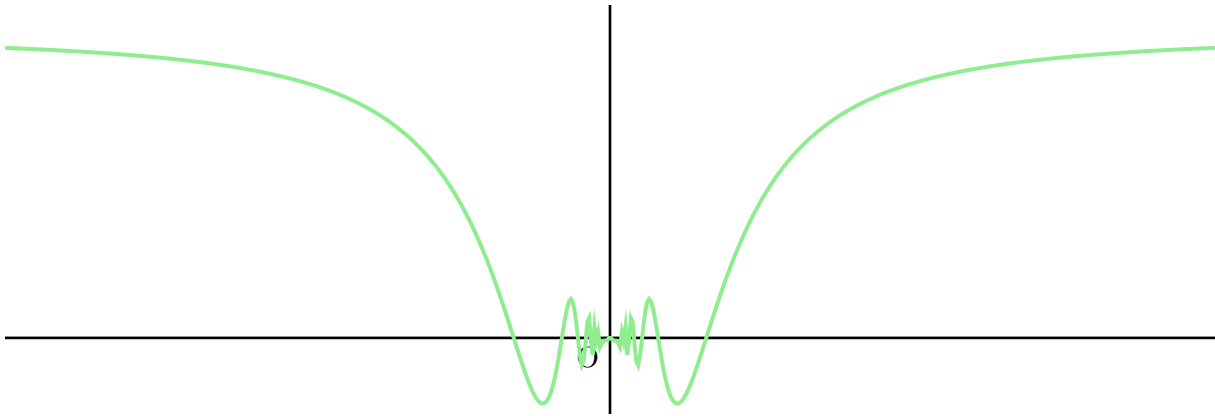
Figure XVI.4 – Une fonction peut être continue sans être dérivable ni à gauche, ni à droite.
