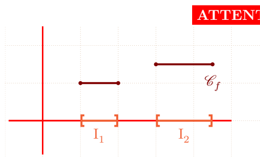
Figure XVI.11 – f est constante sur I_1 et I_2 mais n'est pas constante sur I = I_1 \cup I_2 .
