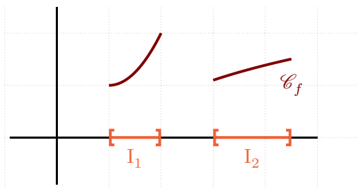
Figure XVI.12 – f est croissante sur I_1 et I_2 donc f' \geq 0 mais n'est pas croissante sur I = I_1 \cup I_2 .
