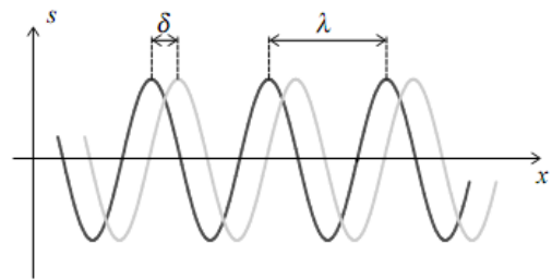
Figure 2.14 – Onde sinusoïdale se propageant dans le sens positif de (Ox) à deux instants t_0 (en gris foncé) et t_1 > t_0 (en gris clair).
