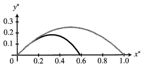
Figure 15.16 – Comparaison entre une trajectoire avec frottement pour laquelle v_0 = v_l (en noir) et une trajectoire sans frottement avec la même vitesse initiale (en gris). Les frottements diminuent la portée sans changer fondamentalement la forme de la trajectoire. L'angle de tir est de 45^\circ par rapport à l'horizontale.
