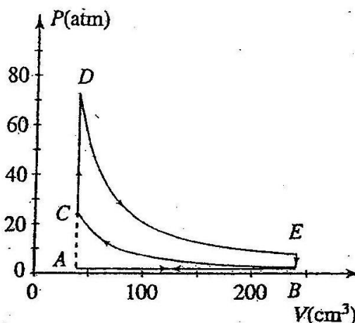
Doc 9. Diagramme de Watt d'un cylindre
