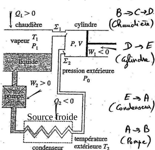
Doc. 1. Schéma de la machine à vapeur de Watt.
