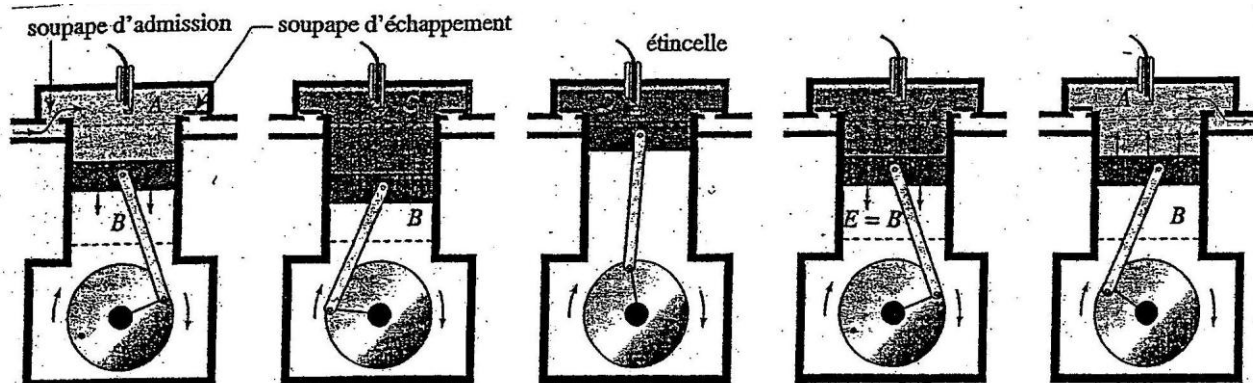
Doc. a. Admission. Doc. b. Compression. Doc. c. Combustion. Doc. d. Détente. Doc. e. Échappement.
