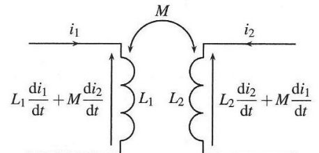
Figure 29.7 – Circuits électriques équivalents (convention récepteur).
