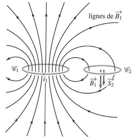
Figure 29.5 – Deux circuits magnétiquement couplés.
