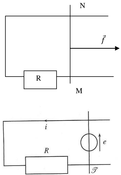
Figure 30.3 – Schéma électrique équivalent.
