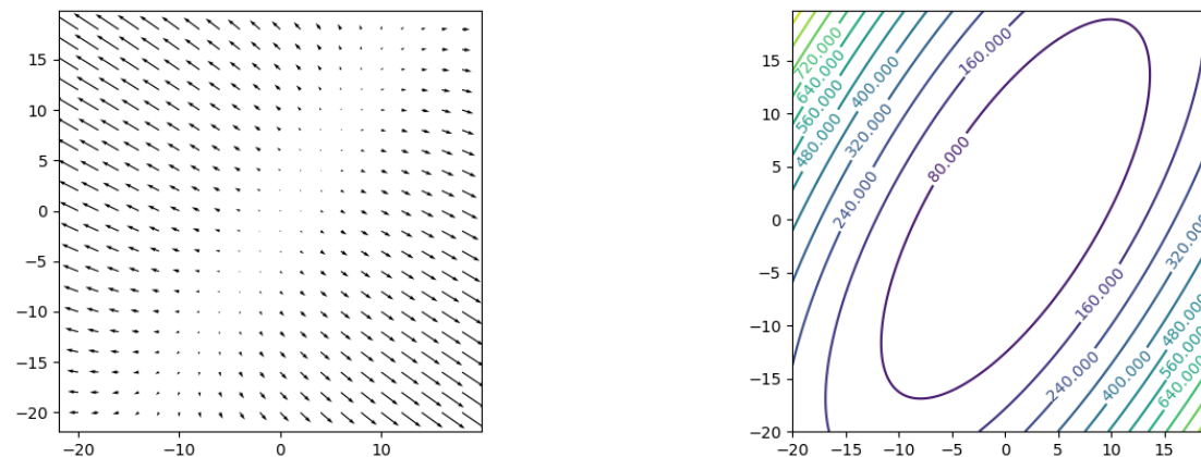
FIGURE 3 – Lignes de niveau et gradient pour (x, y) \mapsto x^2 - y \cdot x
