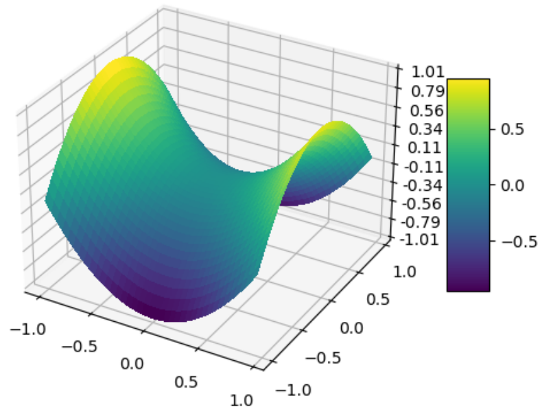
FIGURE 1 – Graphe de la fonction (x, y) \mapsto x^2 - y^2 .
