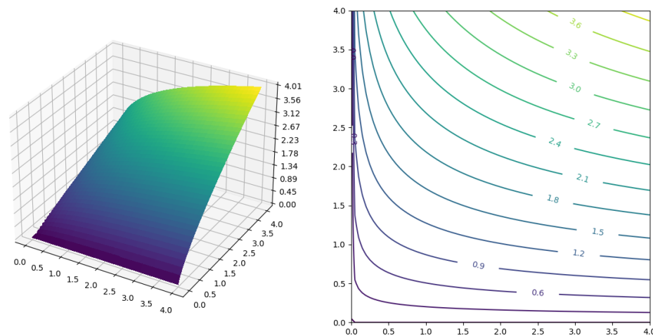
FIGURE 2 – La surface représentative d'une fonction et les lignes de niveaux.
