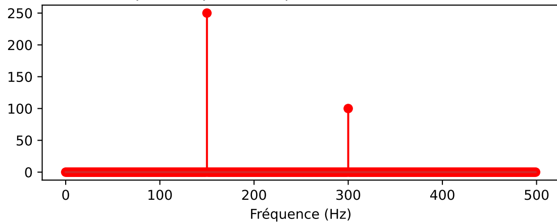
Spectre après filtre passe-haut (fc=100 Hz)
