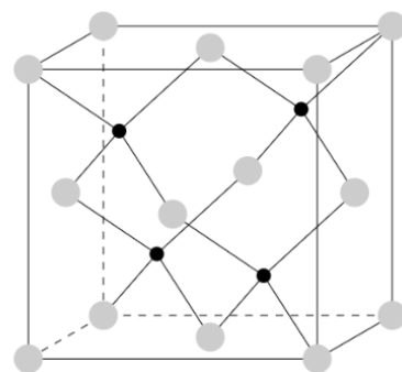
Figure 1 Maille conventionnelle du \beta -SiC
