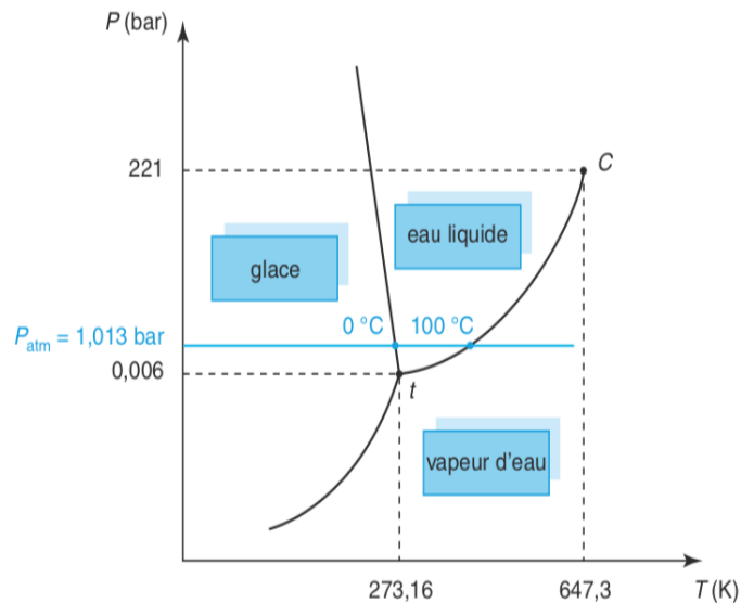
Diagramme d'état (P, T) de l'eau
