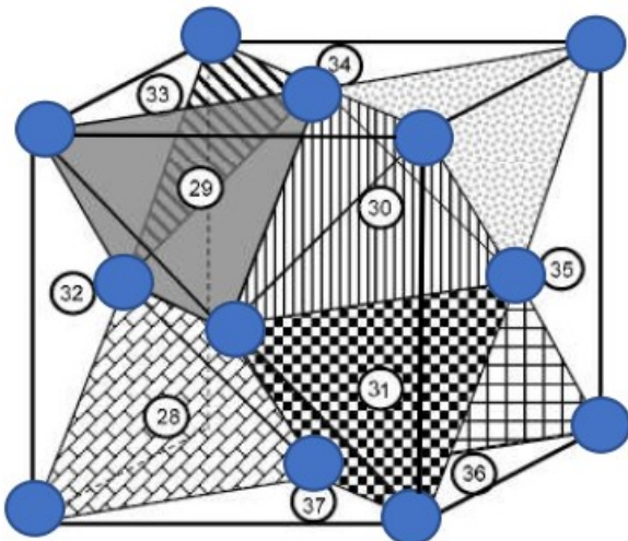
Figure 2b : Structure cubique faces centrées avec représentation des tétraèdres.
