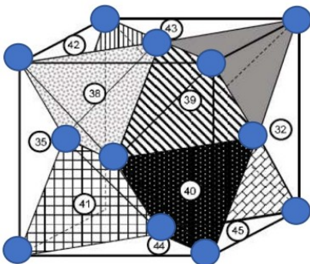
Figure 2c : Rotation de 180° de la figure 2b .
