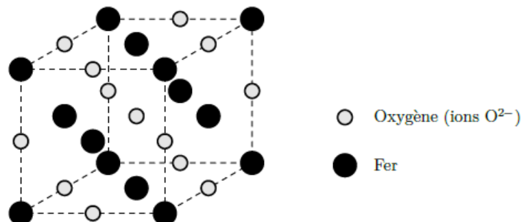
FIGURE 2 – Structure cristalline de l'oxyde ferreux
