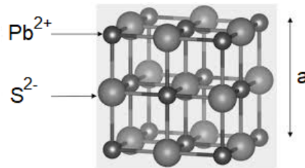
FIGURE 3 – Maille du cristal de sulfure de plomb
