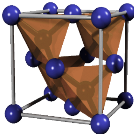
FIGURE 5 – Représentation d'une maille cristalline du diamant
