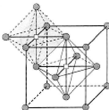
FIGURE 4 – Représentation du site octaédrique central et d'un site octaédrique latéral dans la maille cubique à faces centrées
