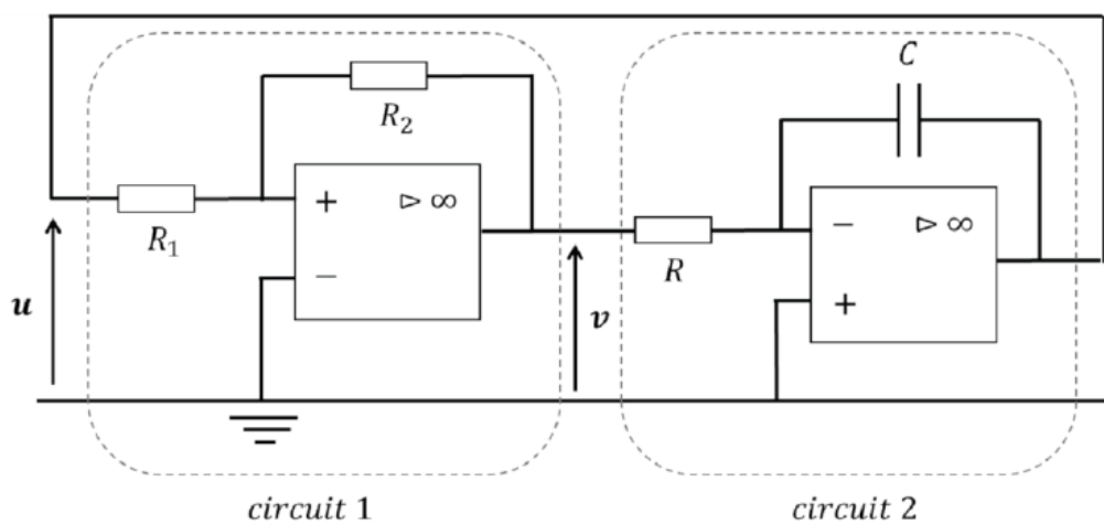
Document 1 : exemple d'oscillateur à relaxation
