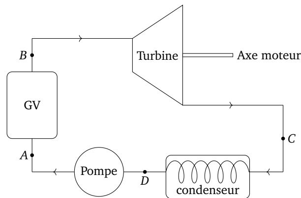
Figure 2 – Cycle de Rankine étudié
