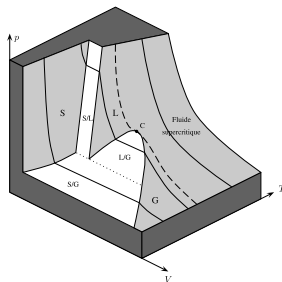
Diagramme p-V-T
