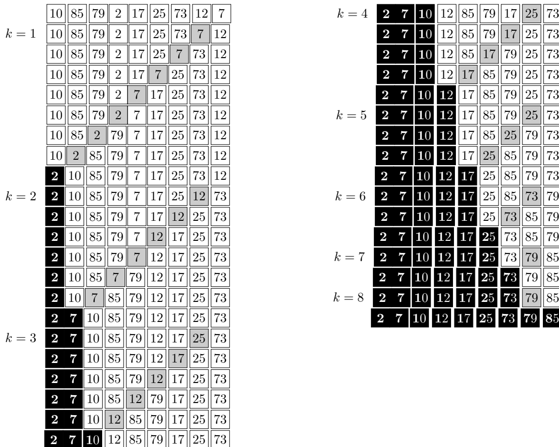
FIGURE 1 – Fonctionnement du tri à bulles avec la séquence [10, 85, 79, 2, 17, 25, 73, 12, 7]. À chaque itération k \in \llbracket 1, 8 \rrbracket , la case grise représente le résultat de la comparaison des couples, en noir la portion de séquence déjà triée.
