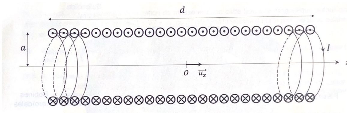
FIGURE 1 – Schéma du solénoïde. Seules quelques spires sont représentées par souci de lisibilité.
