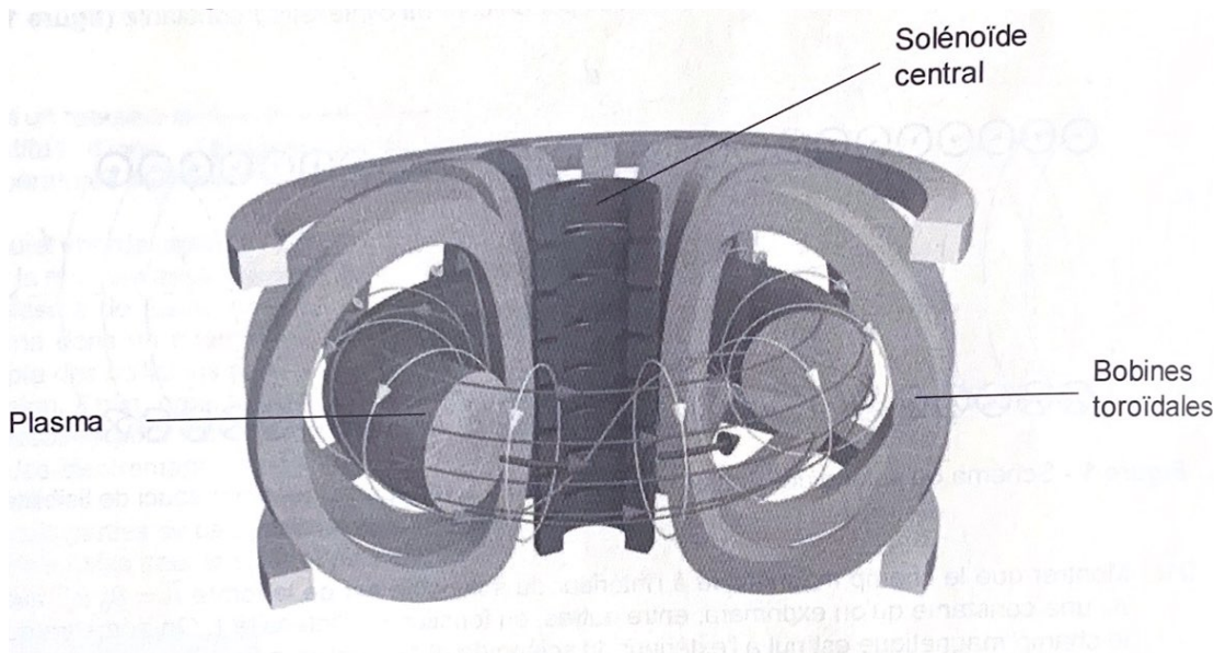
FIGURE 2 – Schéma d'un tokamak
