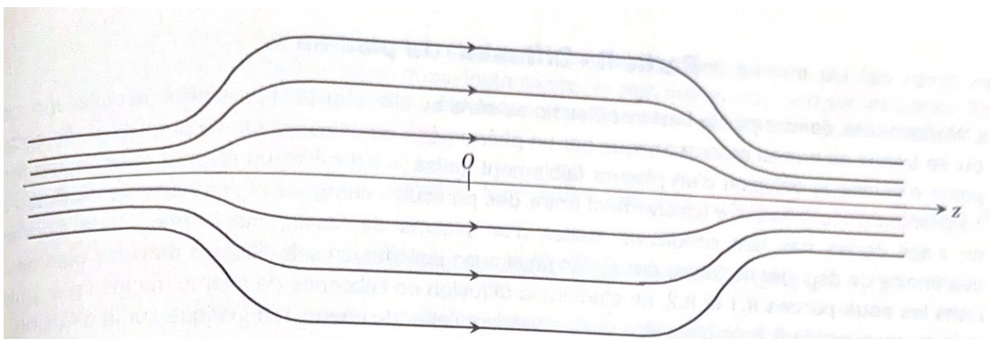
FIGURE 3 – Lignes de champ d'une bouteille magnétique
