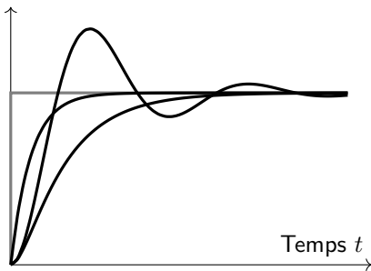
Systèmes stables
