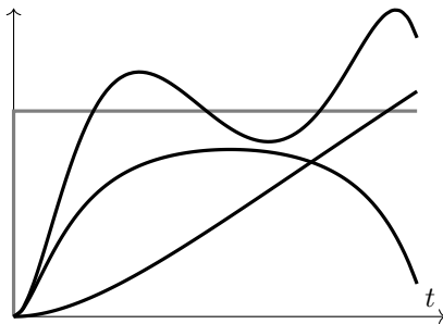
Systèmes instables
